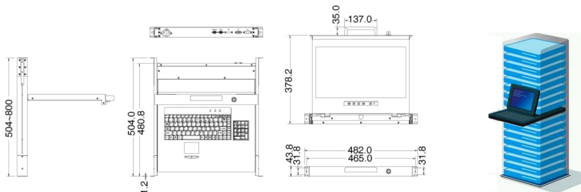
PSR-17HD 寸法図
